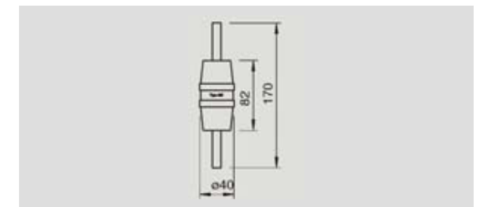
481尺寸图
